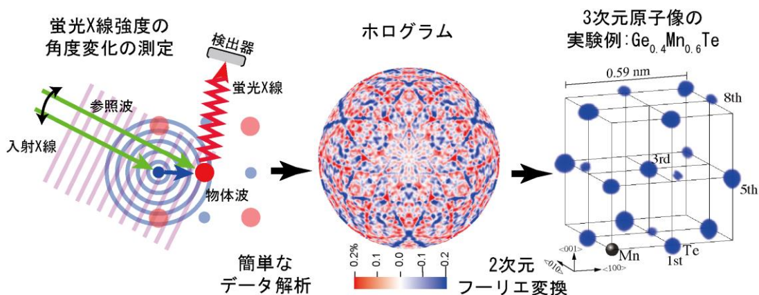
図6 蛍光X線ホログラフイー(XFH)の原理
