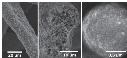
図2 綿形状人工骨を構成する繊維状複合材料の走査型電子顕微鏡写真。(左) 繊維の形状: 幅50μm程度、厚さ10~20μmの扁平状の長繊維であり、骨形成性細胞の接着・増殖に適した面積が確保されている。(中) 繊維の断面: 生分解性ポリマーマトリックス中に微細なセラミック粒子が充填された複合体である。(右) セラミック微粒子の拡大像: 10~20nmの炭酸カルシウムナノ粒子が凝集して直径1~2μmの球状粒子が形成されている。ケイ素成分が2.5%含まれており、生体内埋植後に優先的に溶解して骨形成を促進する効果を引きだす。
